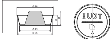
86/8BB - Зашт. поклопац
