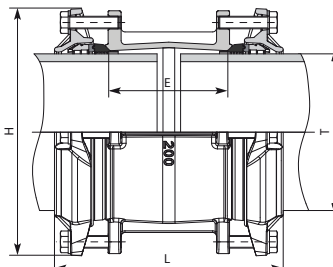
екст. Ø160 и Ø200
