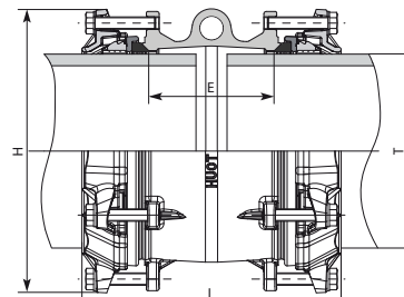
екст. Ø225 до Ø315
