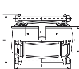
екст. Ø40 до Ø140
